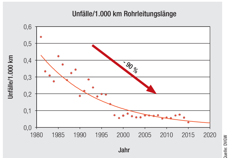
Abb. 5: Zeitliche Entwicklung von Unfällen an Gasrohrleitungen in Deutschland: Seit 1980 ist die Unfallrate um 90 % gesunken.
