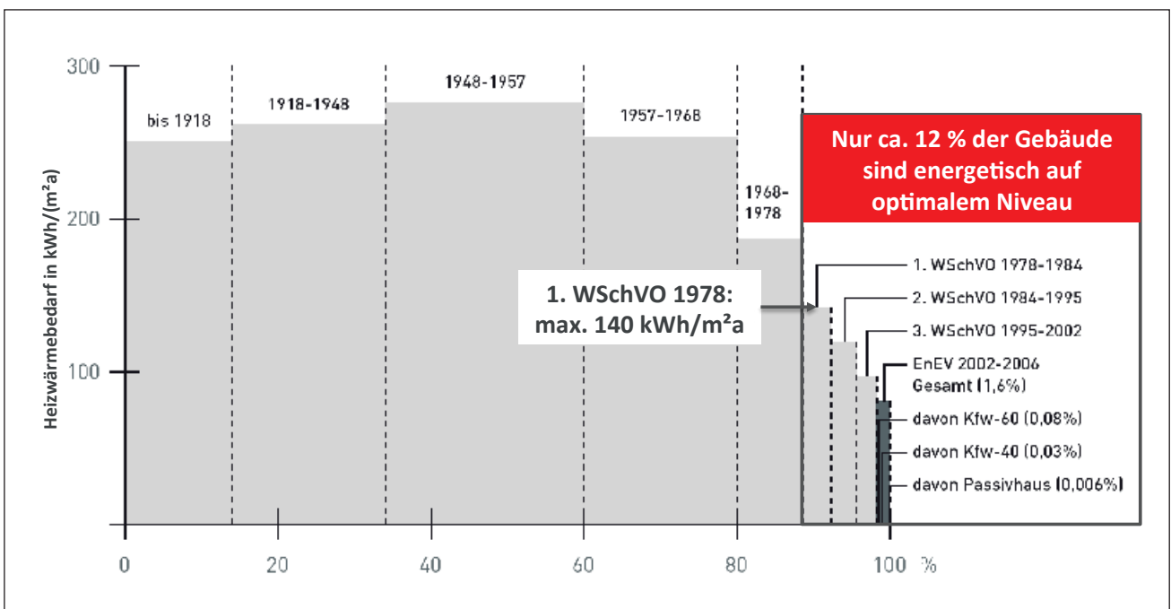
Abb. 4: Heizwärmebedarf von Gebäuden. Die Energiewende im Wärmemarkt findet im Bestand statt.
