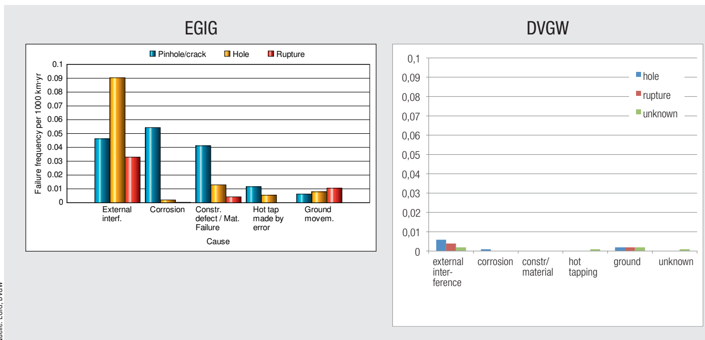
Abb. 6: Vergleich EGIG - DVGW Unfälle in Abhängigkeit der Ursachen (1.000 km * Jahr)
