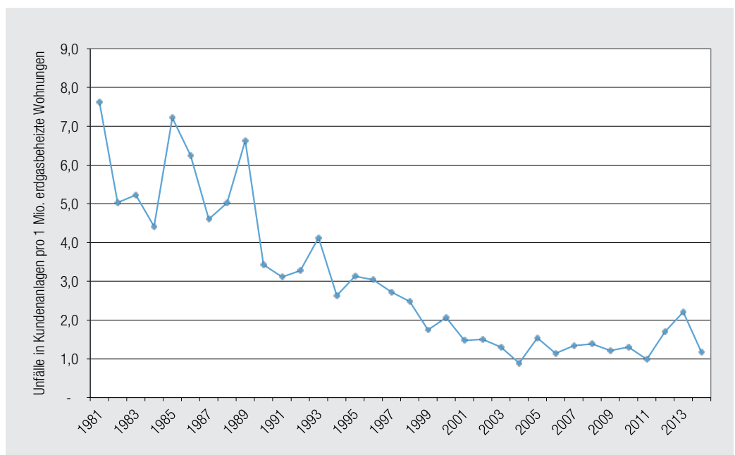
Abb. 7: Rückgang der Unfälle an Kundenanlagen seit 1981
